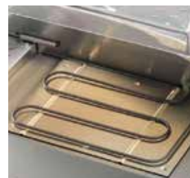
Os modelos Dry utilizam uma bateria de resistências situadas na parte inferior da cuba.
